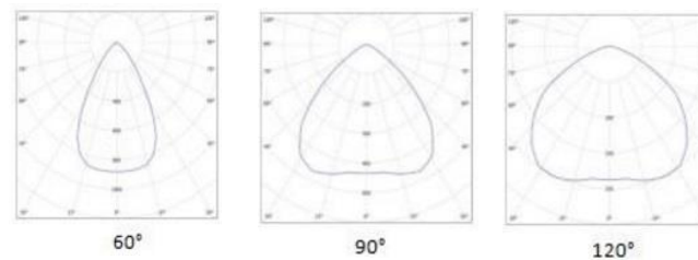
Vyzařovací charakteristika
